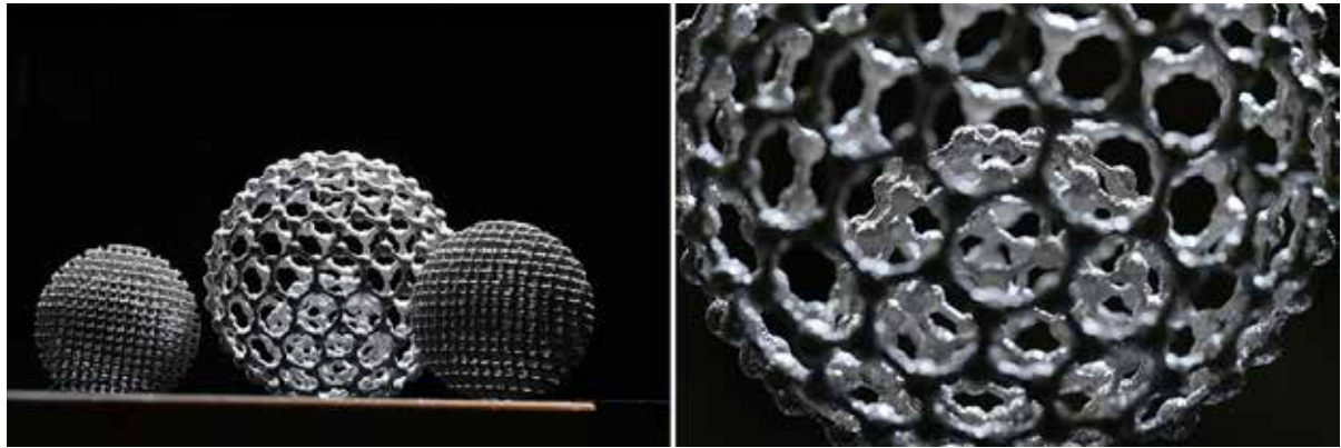
写真7 造形品のサンプル（左）。中央の網球状の造形物には同様の造形物が内包されている（右）。造形物の中に別の造形物を一度の工程で作製できることも、この3Dプリンターならではの特長
