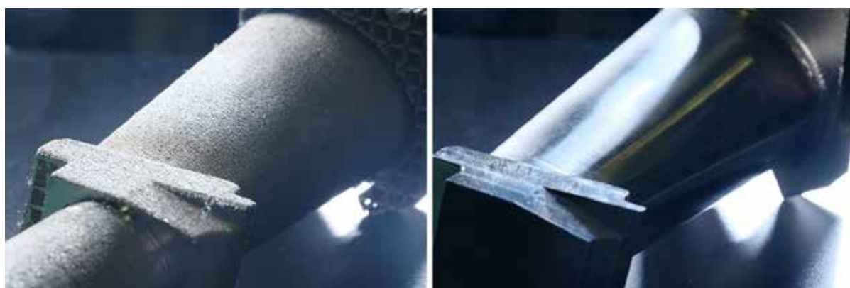
写真 10 仮焼結した金属粉末を除去中の発電用のタービンブレード (左) と、除去後、磨きだして完成したもの (右)
