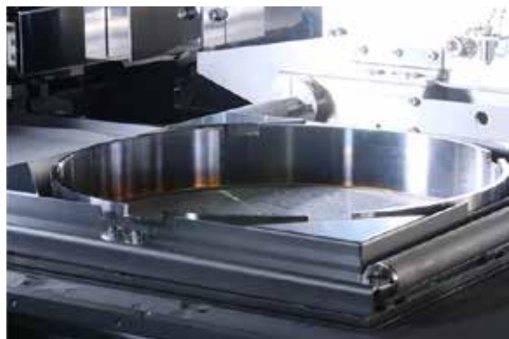
写真2 チャンバー内に、積層造形スペースを囲うように設置された「e-Shield」
