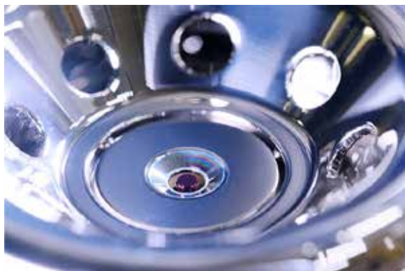
写真 5 「JAM-5200EBM」の電子銃ビーム照射口
