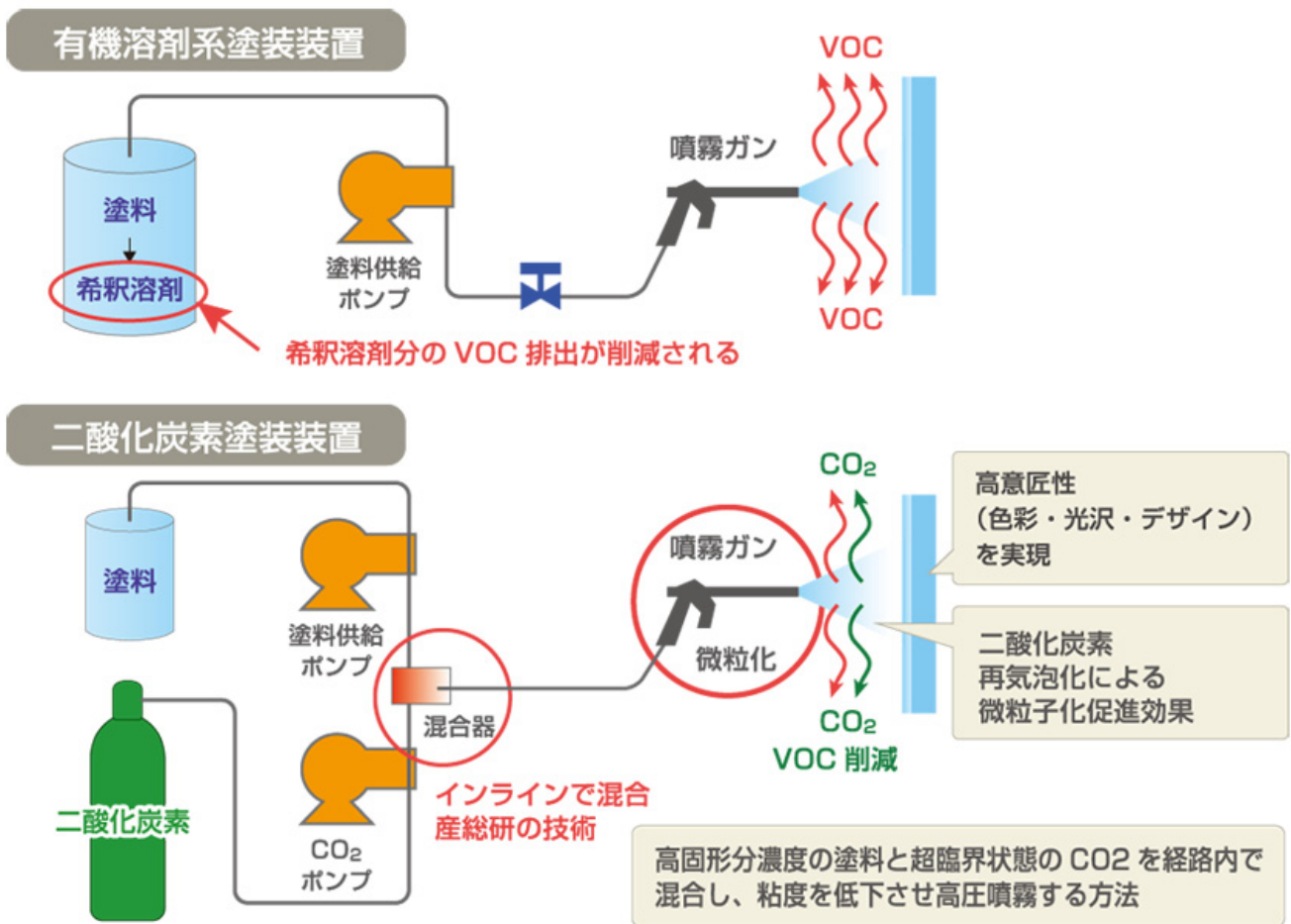
図5 有機溶剤塗装と二酸化炭素塗装の違い。混合器と噴霧ガンノズルの開発がポイントだった
