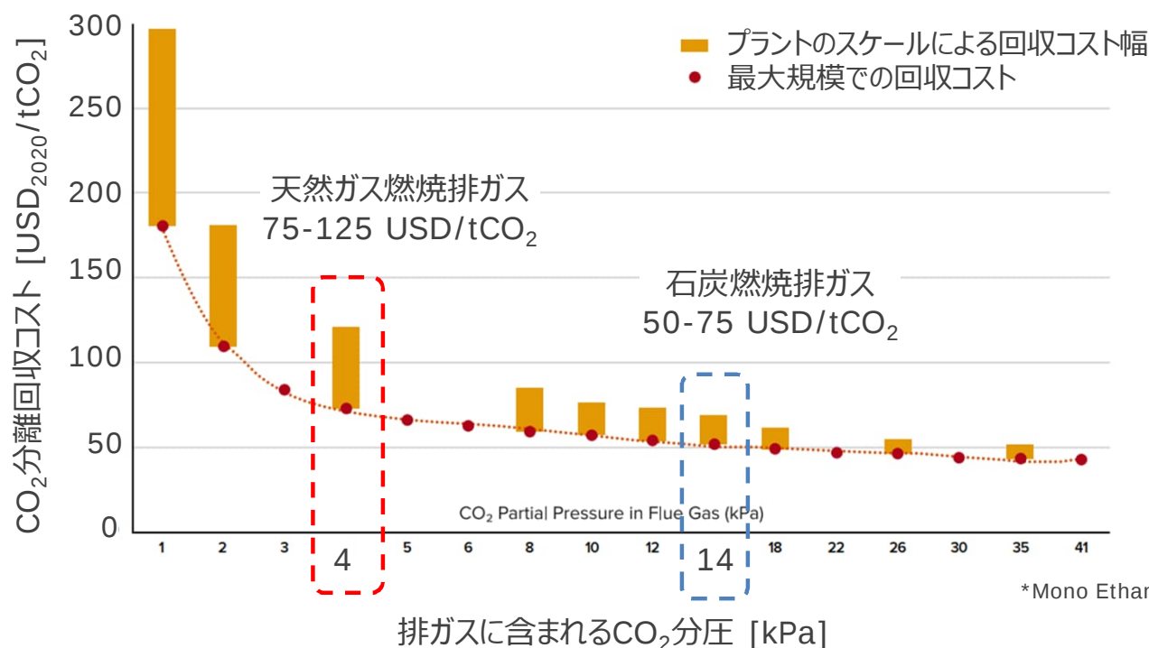
30%モノエタノールアミン液を用いた際のCO 2 回収コスト試算
