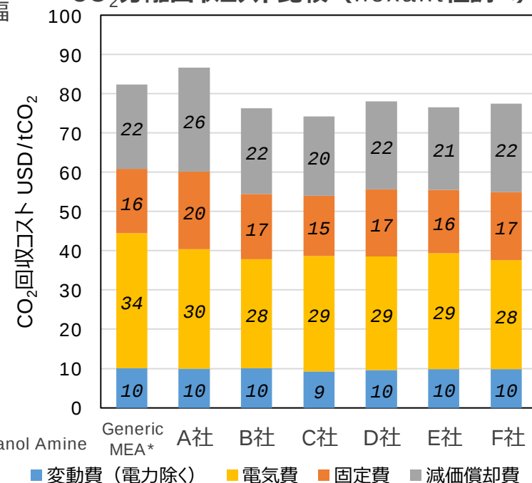
アミン吸収液法によるNGCCからのCO 2 分離回収コスト比較 (nexant社調べ)
