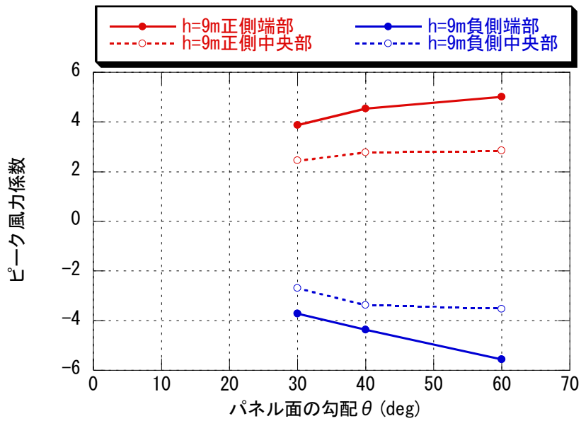
図 6-7 領域別パネルの面平均最大・最小ピーク風力係数 ( h=9\text{m} 、パネル角度 \theta による比較)
