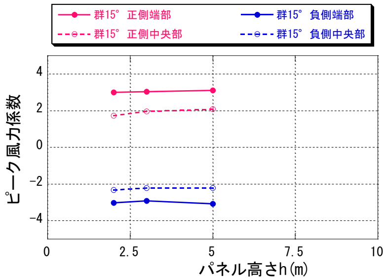
図 6-9 領域別パネルの面平均最大・最小ピーク風力係数 ( \theta=15^\circ 、パネル高さ h による比較)
