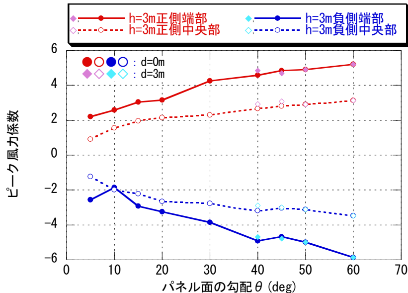
図 6-5 領域別パネルの面平均最大・最小ピーク風力係数 ( h=3\text{m} 、パネル角度 \theta による比較)
