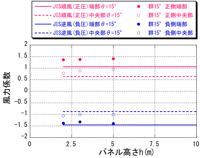
図 6-23 領域別パネルの面平均最大・最小風力係数 (JIS 値との比較) ( \theta=15^\circ 、パネル高さ h による比較)
