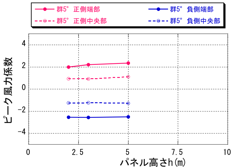
図 6-8 領域別パネルの面平均最大・最小ピーク風力係数 ( \theta=5^\circ 、パネル高さ h による比較)
