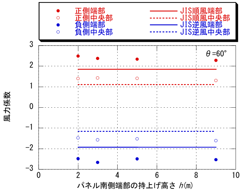
図 6-28 領域別パネルの面平均最大・最小風力係数（JIS 値との比較） (\theta=60^\circ 、パネル高さ h による比較)
