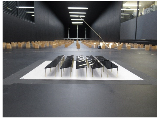
(d) m10h3(h=3m , \theta = 10^\circ )
