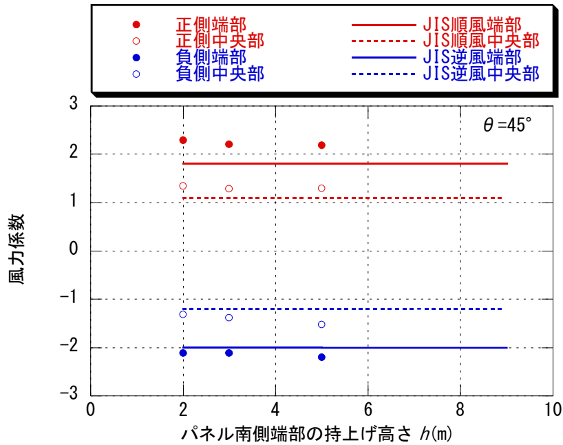
図 6-26 領域別パネルの面平均最大・最小風力係数 (JIS 値との比較) ( \theta=45^\circ 、パネル高さ h による比較)
