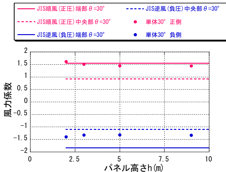
図 6-17 単体パネルの面平均最大・最小風力係数（JIS 値との比較） ( \theta=30^\circ 、パネル高さ h による比較)
