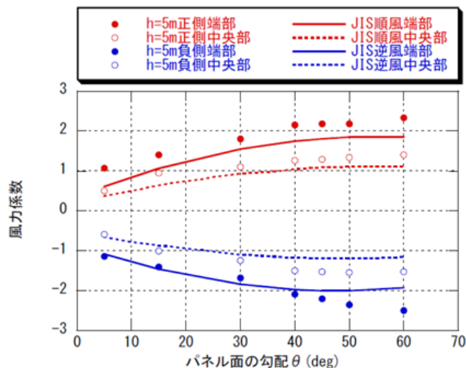
図 6-20 領域別パネルの面平均最大・最小風力係数（JIS 値との比較） ( h=5\text{m} 、パネル角度 \theta による比較)
