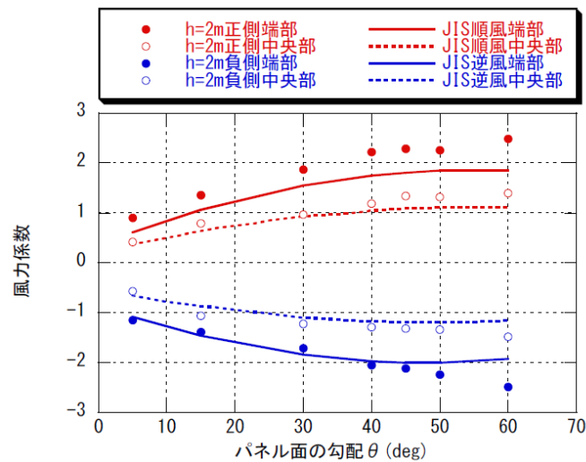
図 6-18 領域別パネルの面平均最大・最小風力係数（JIS 値との比較） ( h=2\text{m} 、パネル角度 \theta による比較)
