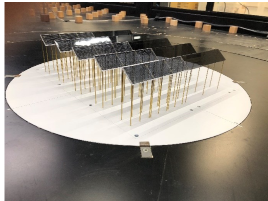
(e) m40h9(h=9m, \theta = 40 度)
