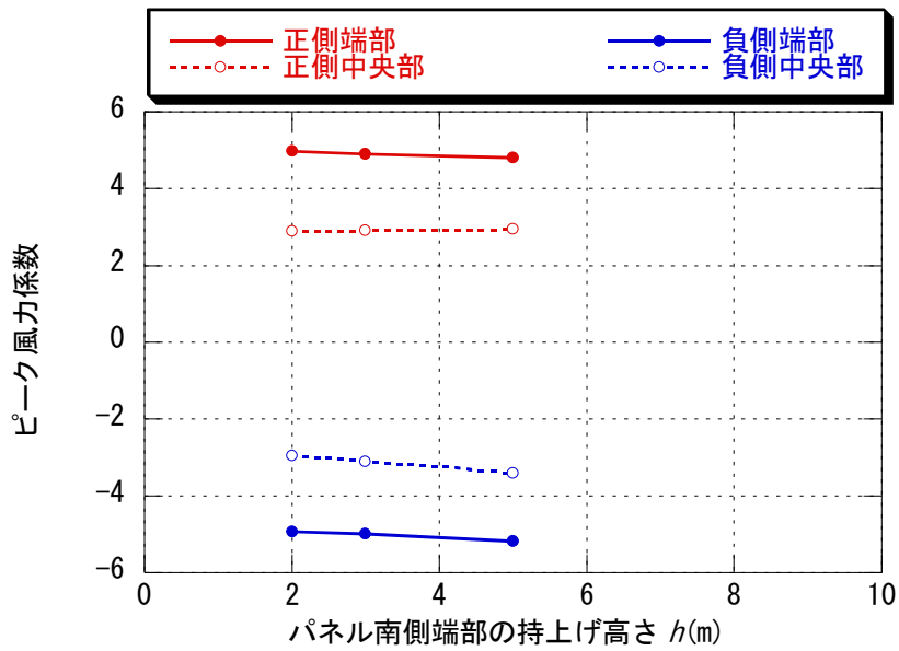
図 6-13 領域別パネルの面平均最大・最小ピーク風力係数 ( \theta=50^\circ 、パネル高さ h による比較)
