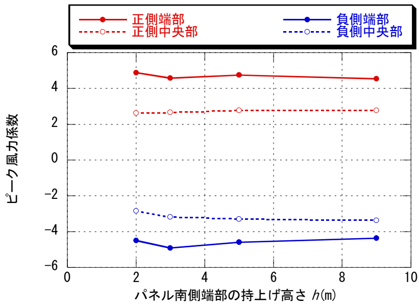
図 6-11 領域別パネルの面平均最大・最小ピーク風力係数 ( \theta=40^\circ 、パネル高さ h による比較)
