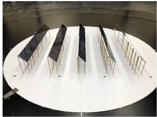
(d) m45h5(h=5m , \theta = 45 度)
