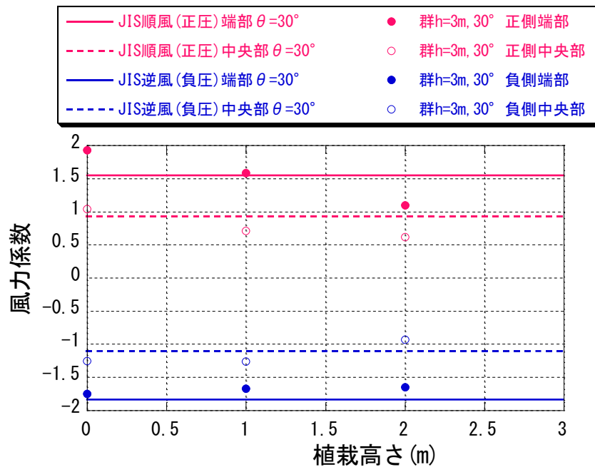
図 6-29 領域別パネルの面平均最大・最小風力係数（JIS 値との比較） (\theta=30^\circ、h=3m、植栽高さによる比較)
