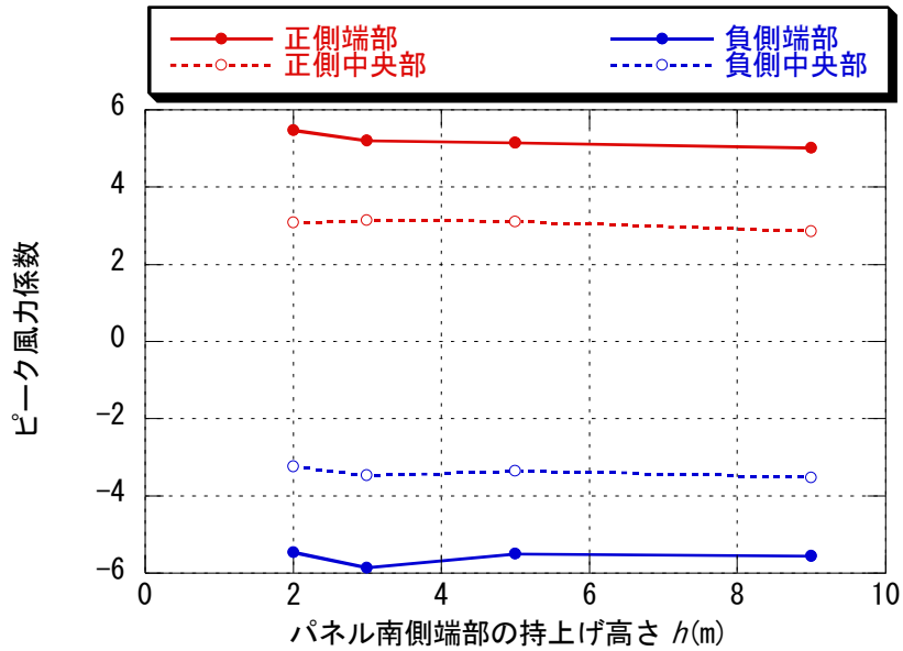
図 6-14 領域別パネルの面平均最大・最小ピーク風力係数 ( \theta=60^\circ 、パネル高さ h による比較)
