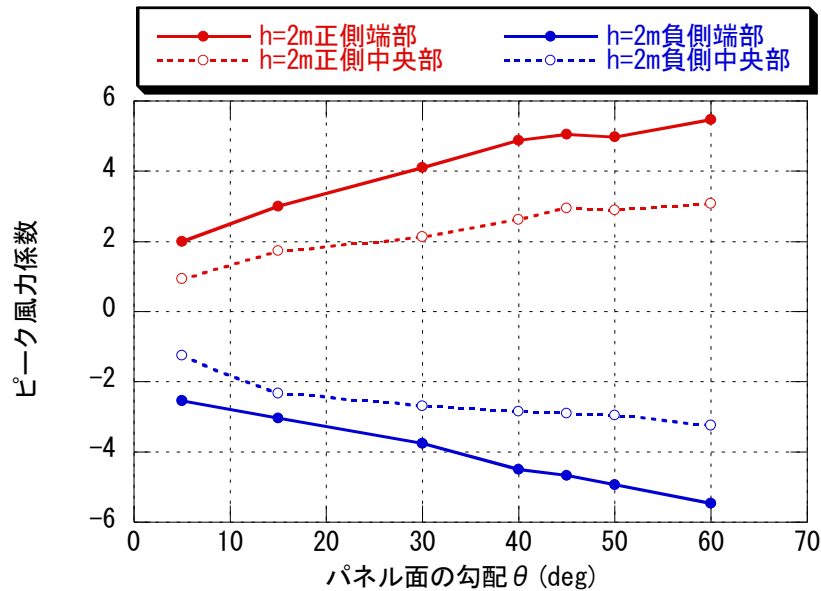
図 6-4 領域別パネルの面平均最大・最小ピーク風力係数 ( h=2\text{m} 、パネル角度 \theta による比較)
