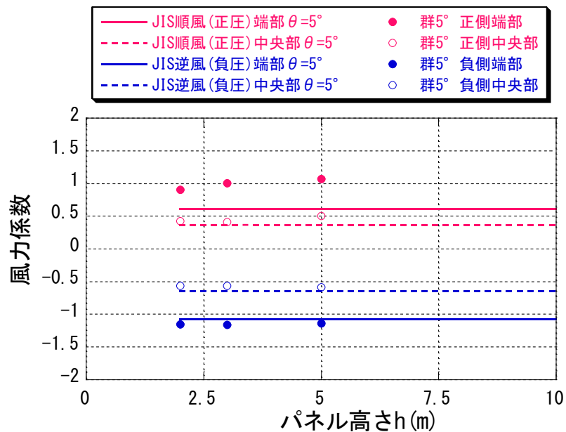
図 6-22 領域別パネルの面平均最大・最小風力係数（JIS 値との比較） ( \theta=5^\circ 、パネル高さ h による比較)
