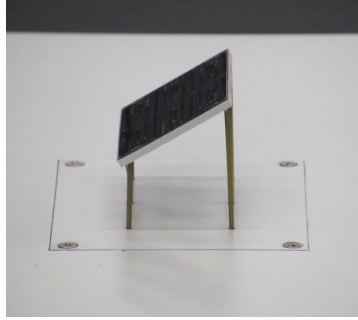
(b) 単体(s30h2)
