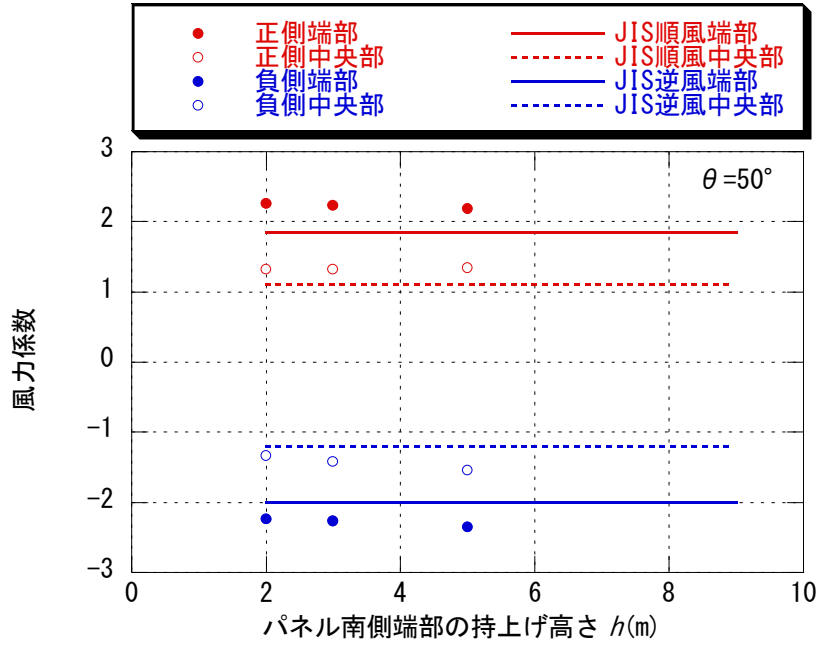
図 6-27 領域別パネルの面平均最大・最小風力係数（JIS 値との比較） (\theta=50^\circ 、パネル高さ h による比較)
