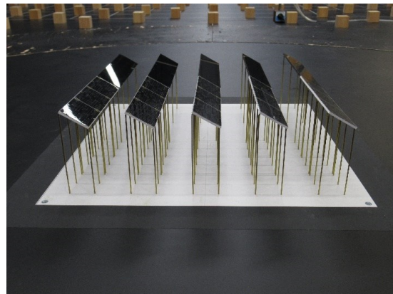
(d) m30h9(h=9m , \theta = 30^\circ )
