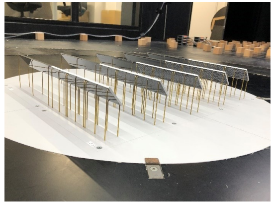
(d) m50h5(h=5m , \theta = 50 度)
