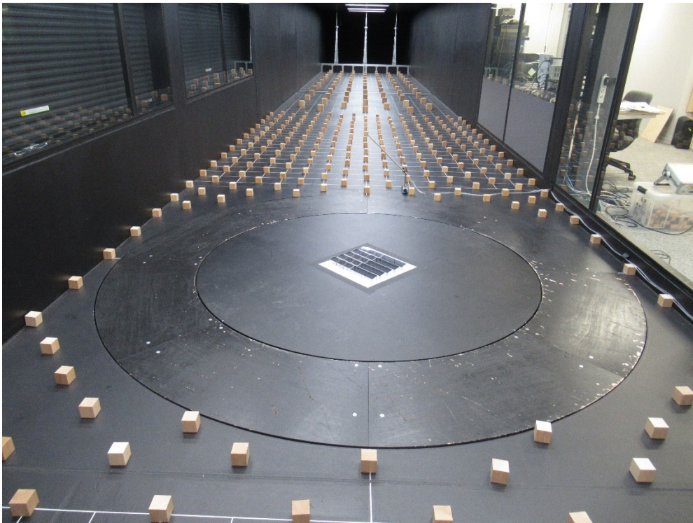
(b) m15h2( h=2\text{m} 、 \theta=15^\circ )
