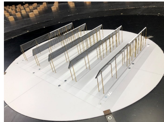
(d) m60h5(h=5m , \theta = 60 度)
