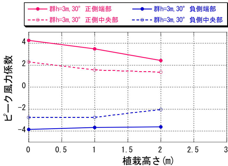
図 6-15 領域別パネルの面平均最大・最小ピーク風力係数 ( \theta=30^\circ 、 h=3\text{m} 、植栽高さによる比較)
