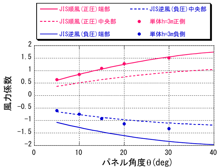
図 6-16 単体パネルの面平均最大・最小風力係数（JIS 値との比較） ( h=3\text{m} 、パネル角度 \theta による比較)
