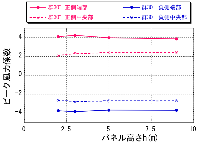
図 6-10 領域別パネルの面平均最大・最小ピーク風力係数 ( \theta=30^\circ 、パネル高さ h による比較)
