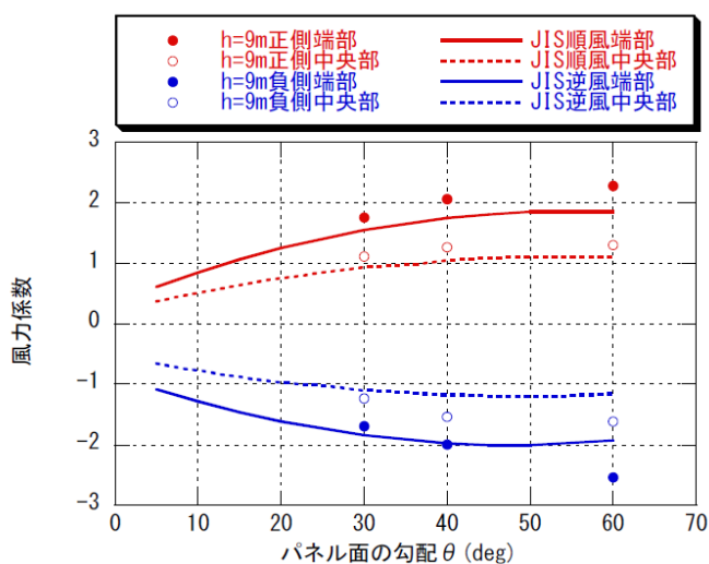
図 6-21 領域別パネルの面平均最大・最小風力係数（JIS 値との比較） ( h=9\text{m} 、パネル角度 \theta による比較)
