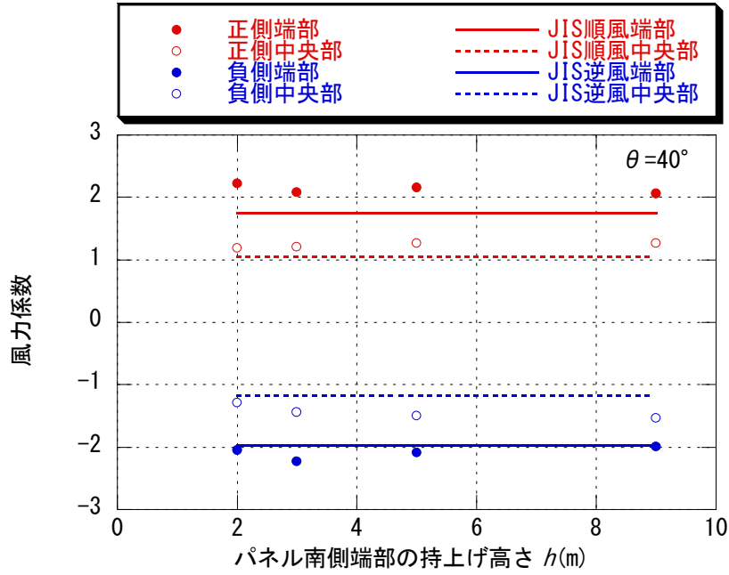
図 6-25 領域別パネルの面平均最大・最小風力係数 (JIS 値との比較) ( \theta=40^\circ 、パネル高さ h による比較)
