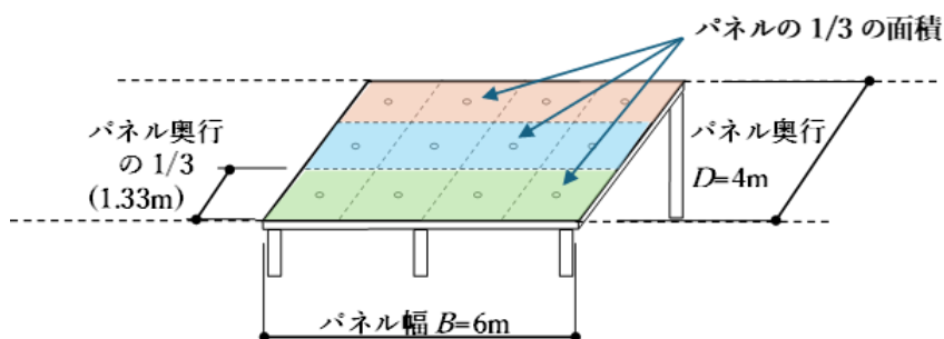
図 8-1 評価対象面積 (パネルの 1/3 の面積)
