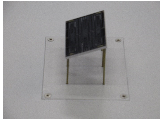
(d) s20h3 ( h=3\text{m} , \theta=20^\circ )
