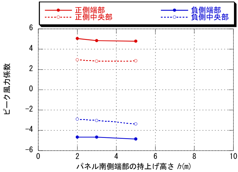
図 6-12 領域別パネルの面平均最大・最小ピーク風力係数 ( \theta=45^\circ 、パネル高さ h による比較)
