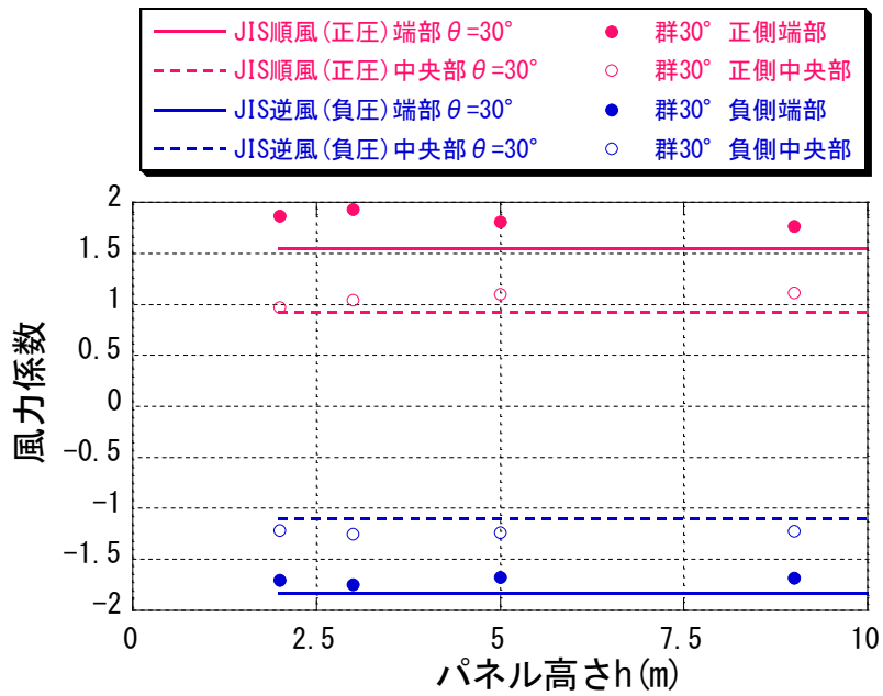
図 6-24 領域別パネルの面平均最大・最小風力係数 (JIS 値との比較) ( \theta=30^\circ 、パネル高さ h による比較)
