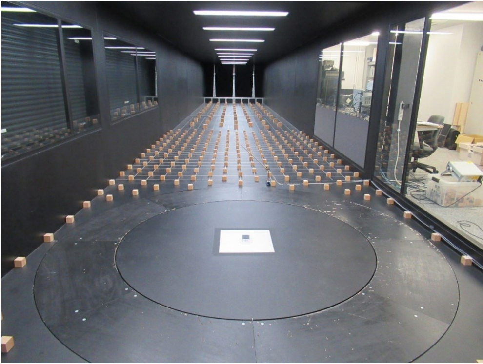
(a) s30h2( h=2\text{m} 、 \theta=30^\circ )
