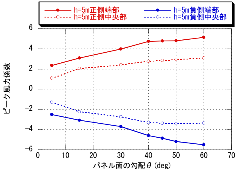
図 6-6 領域別パネルの面平均最大・最小ピーク風力係数 ( h=5\text{m} 、パネル角度 \theta による比較)
