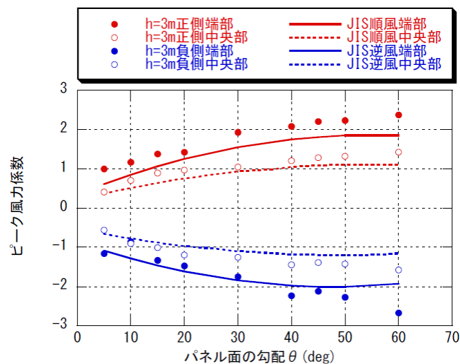
図 6-19 領域別パネルの面平均最大・最小風力係数（JIS 値との比較） ( h=3\text{m} 、パネル角度 \theta による比較)
