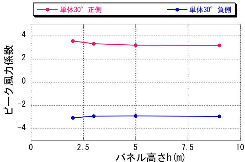
図 6-3 単体パネルの面平均最大・最小ピーク風力係数 ( \theta=30^\circ パネル高さ h による比較)
