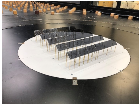
(d) m40h5(h=5m , \theta = 40 度)
