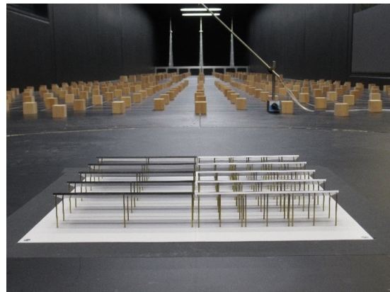
(d) m20h3( h=3\text{m} , \theta =20^\circ )
