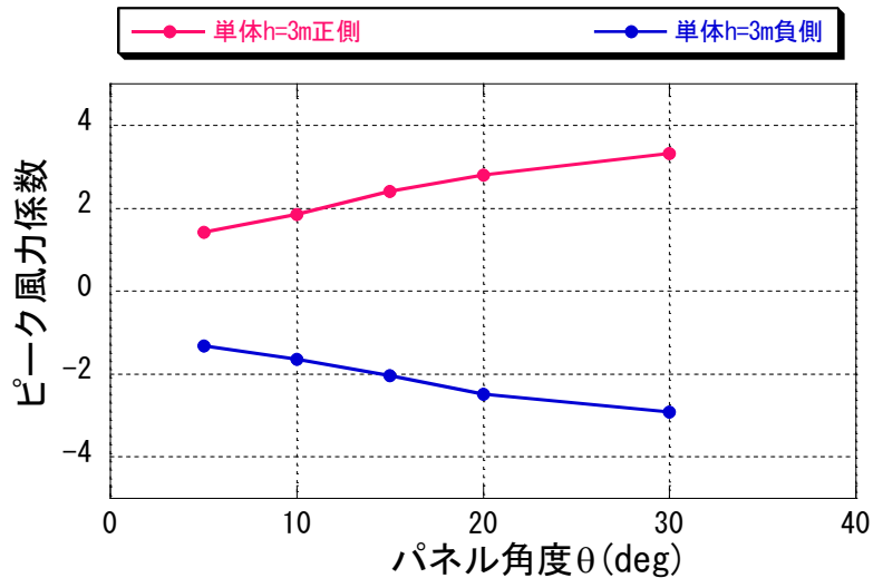
図 6-2 単体パネルの面平均最大・最小ピーク風力係数 ( h=3\text{m} 、パネル角度 \theta による比較)
