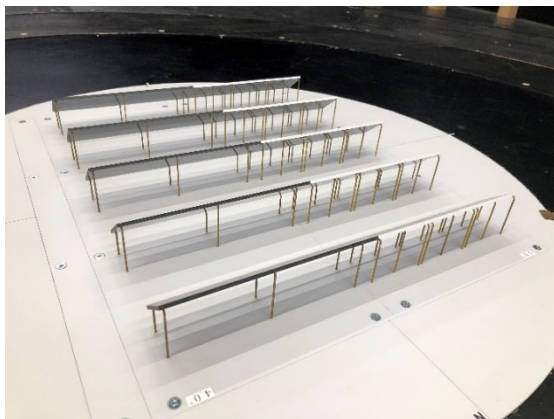
(a) 風圧実験模型 (m40h2)
