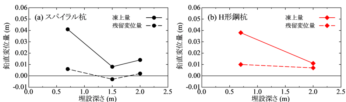
図 3-3 2 種類の杭の埋設深さと凍上量および残留変位量の関係
