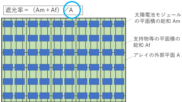
図 6-2 遮光率の定義
