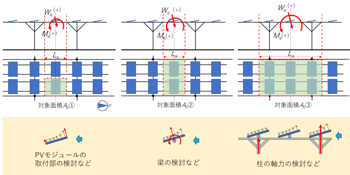
図 7-4 風圧荷重 W_a , M_a , 対象面積 A_a 及びモーメント距離 L_a の定義
