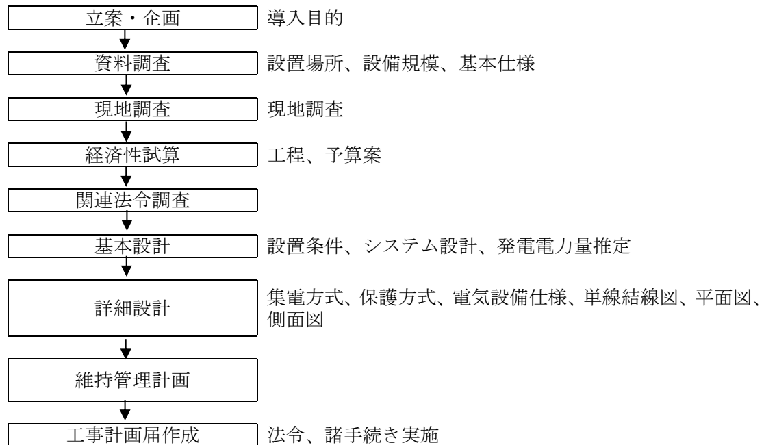
図 4-1 電気設計フロー 4-1)
