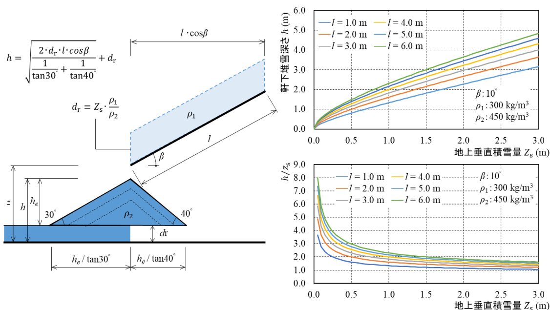
図 7-6 軒高算定モデルと地上垂直積雪量と軒高との関係
