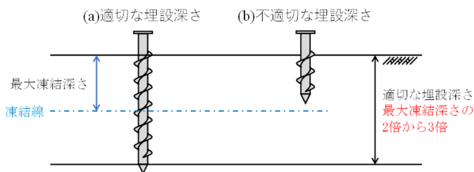
図10-4 杭基礎の適切な埋設方法
