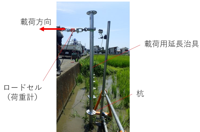
(c) 水平荷重試験の状況
