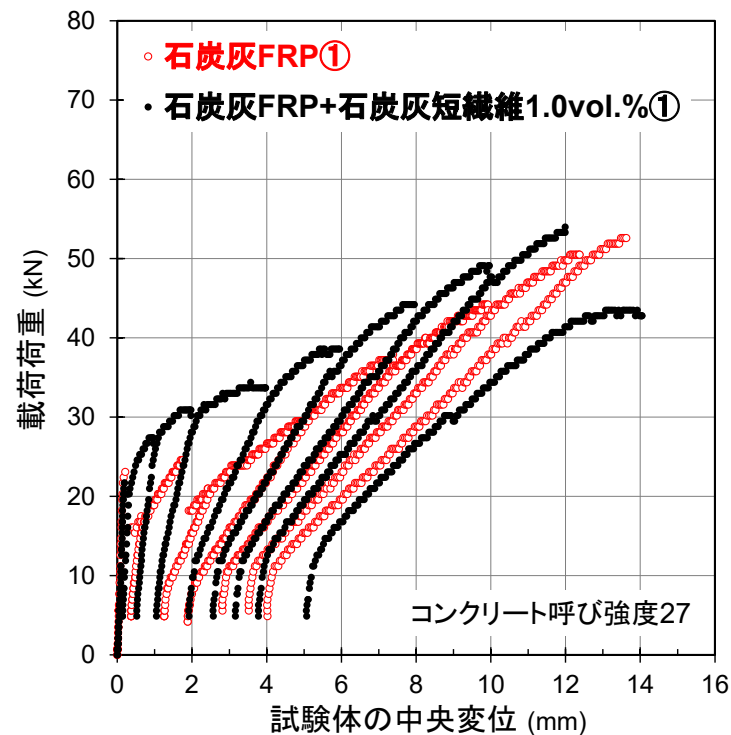
ハイブリッド補強コンクリート 変位-載荷荷重グラフ
