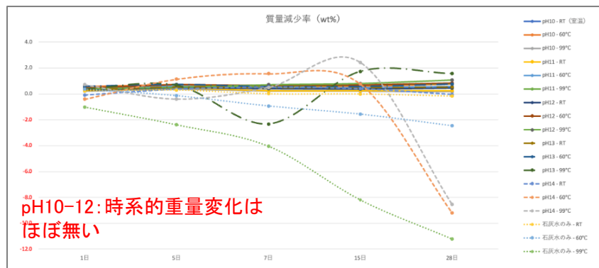
CACLF ロービングに対するNaOH溶液 (pH10~pH14) 及び石灰水への浸漬
