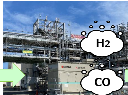
合成ガス製造 (逆シフト反応設備)
