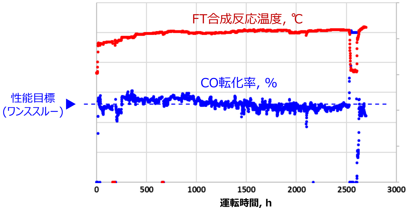
FT合成工程における反応温度・転化率の推移
