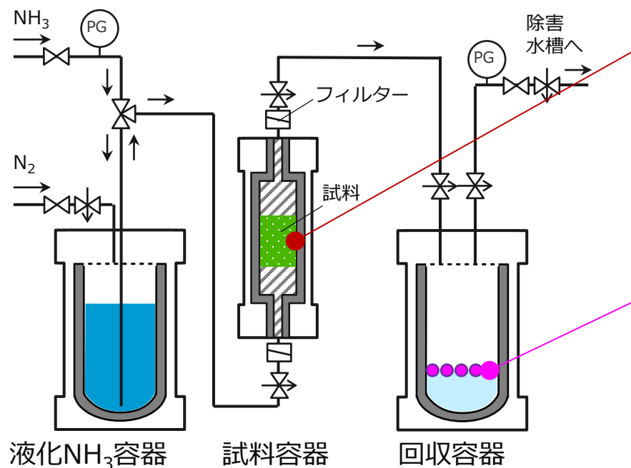
図 液化アンモニアによる抽出試験装置の概略系統
