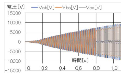
ソフトスタートイメージ [電圧]
