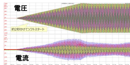
MG蓄電池ソフトスタート時出力
