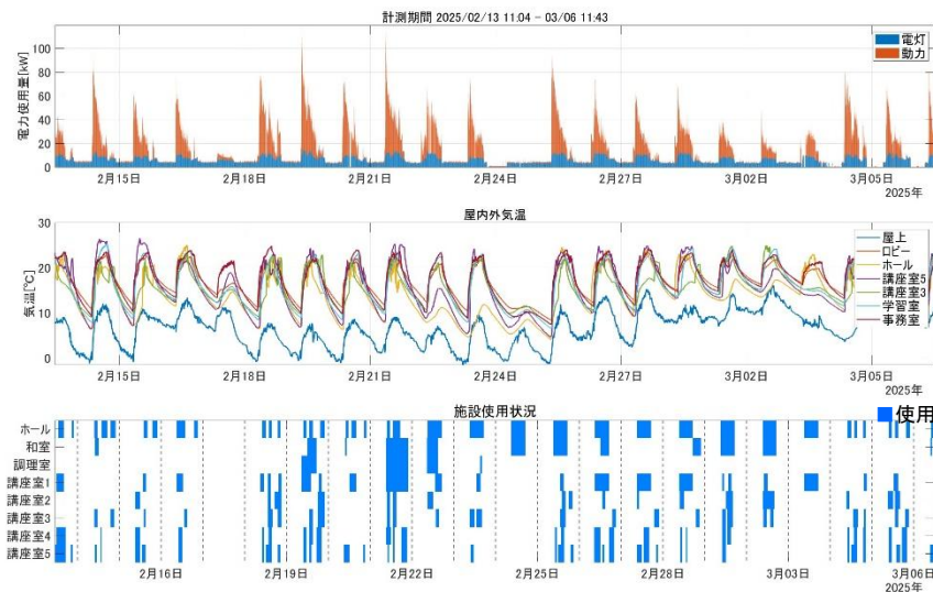
図2 避難所施設(公民館)における冬期の消費電力量・室内温度・設備使用状況の計測結果
