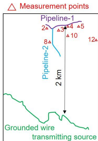
NE-11鋼管と計測点の関係
