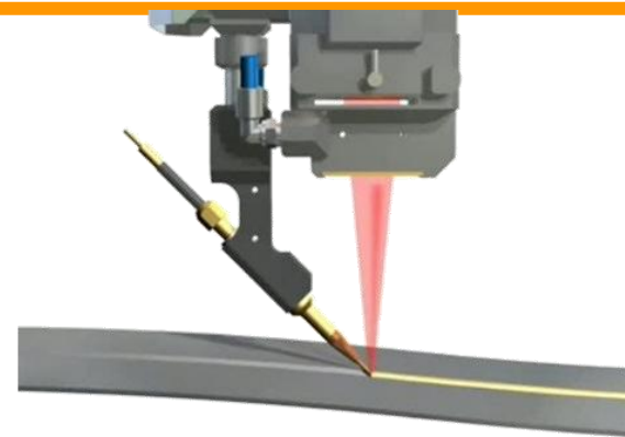
レーザークラディング概略図
