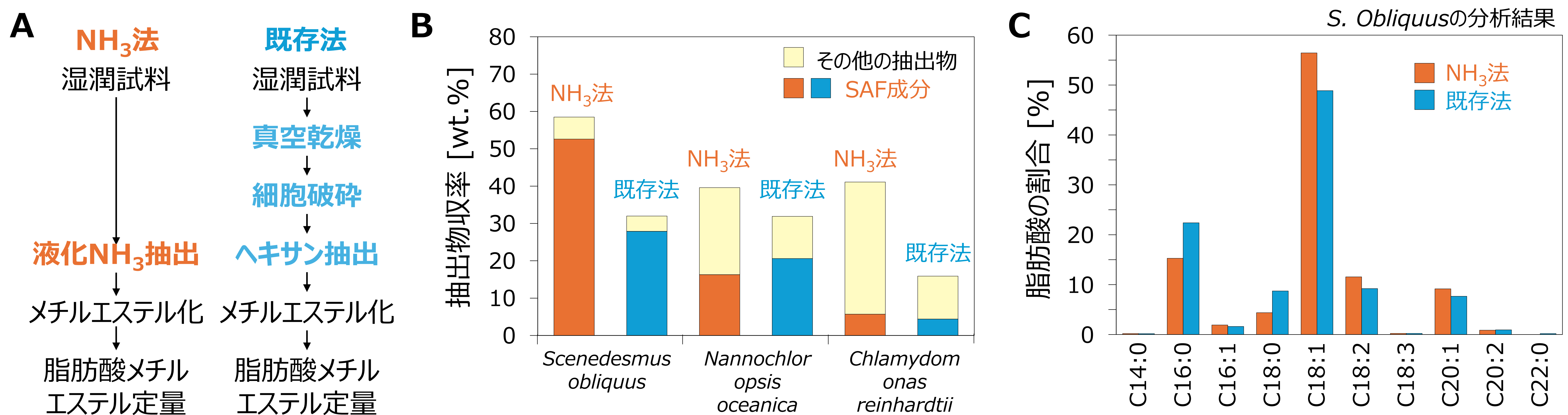
図2 微細藻類からの抽出物収率と脂肪酸組成の分析例
