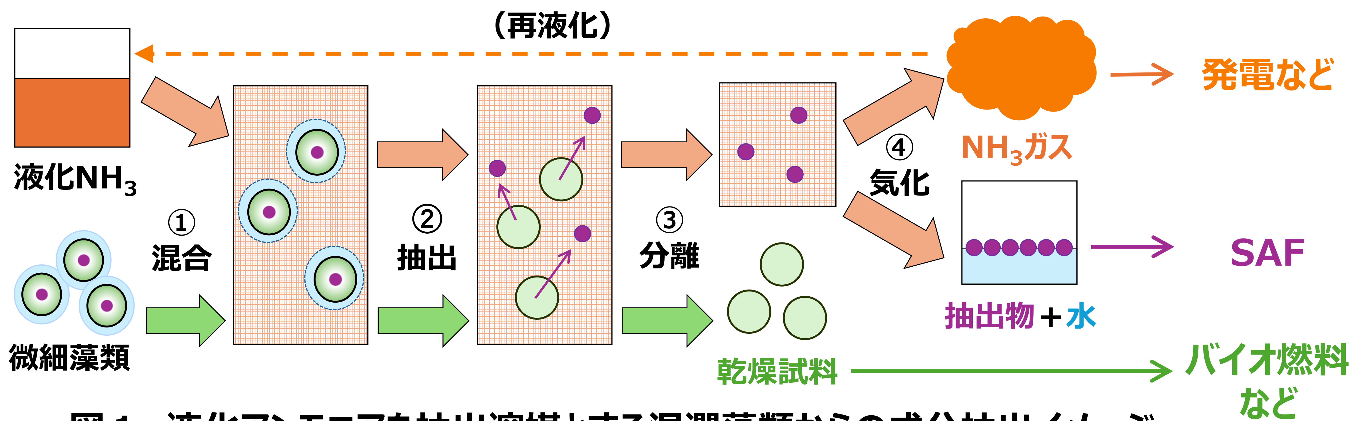
図1 液化アンモニアを抽出溶媒とする湿潤藻類からの成分抽出イメージ
