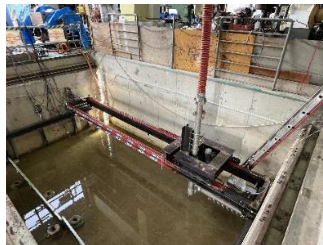
大型土槽実験 (中間スケールでの定量的評価の検証)
