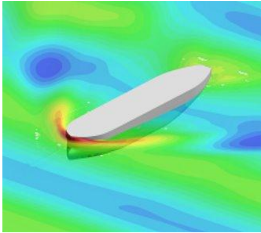
動揺シミュレーションに係るCFD計算イメージ
