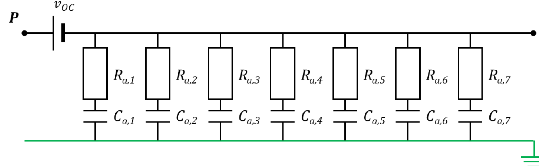
太陽電池モジュール／ストリングの対地等価回路
