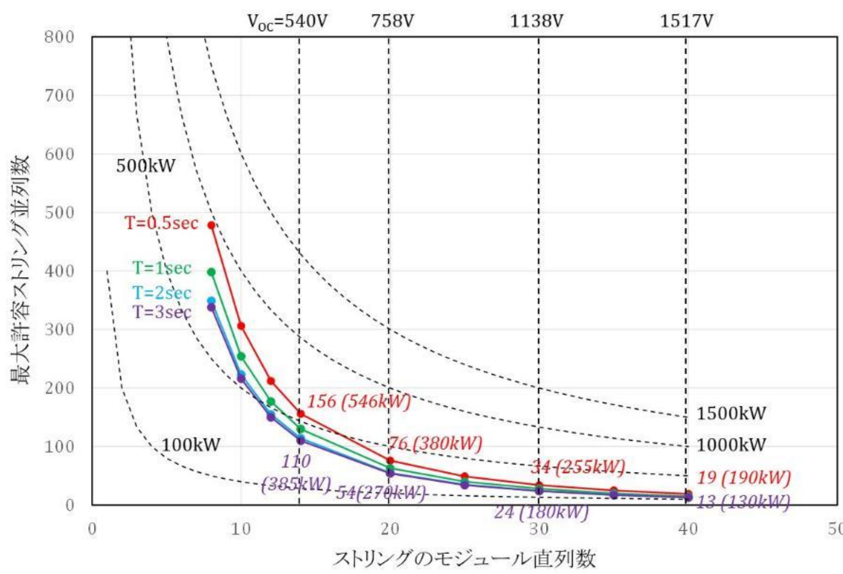
最大許容ストリング並列数の試算例
