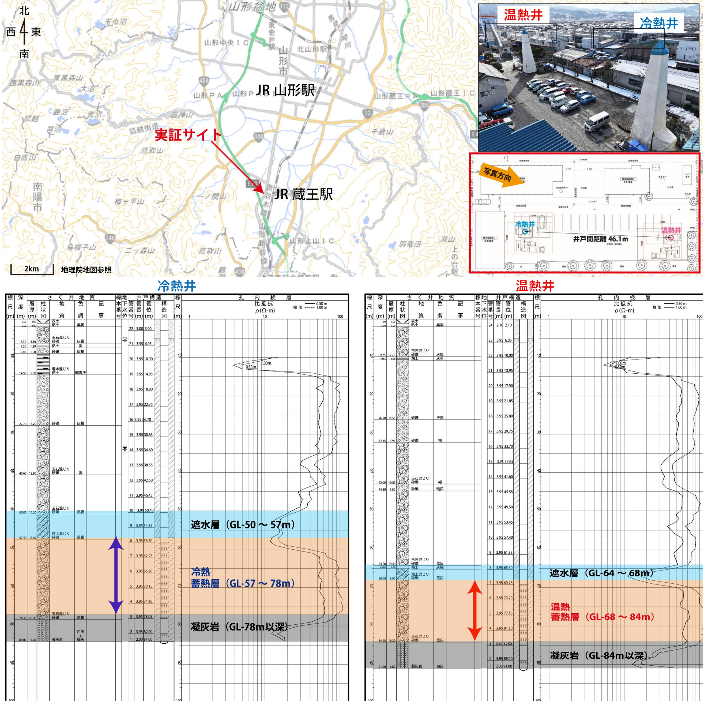
図 実証サイト位置 及び 井戸柱状図(西:冷熱井 東:温熱井)
