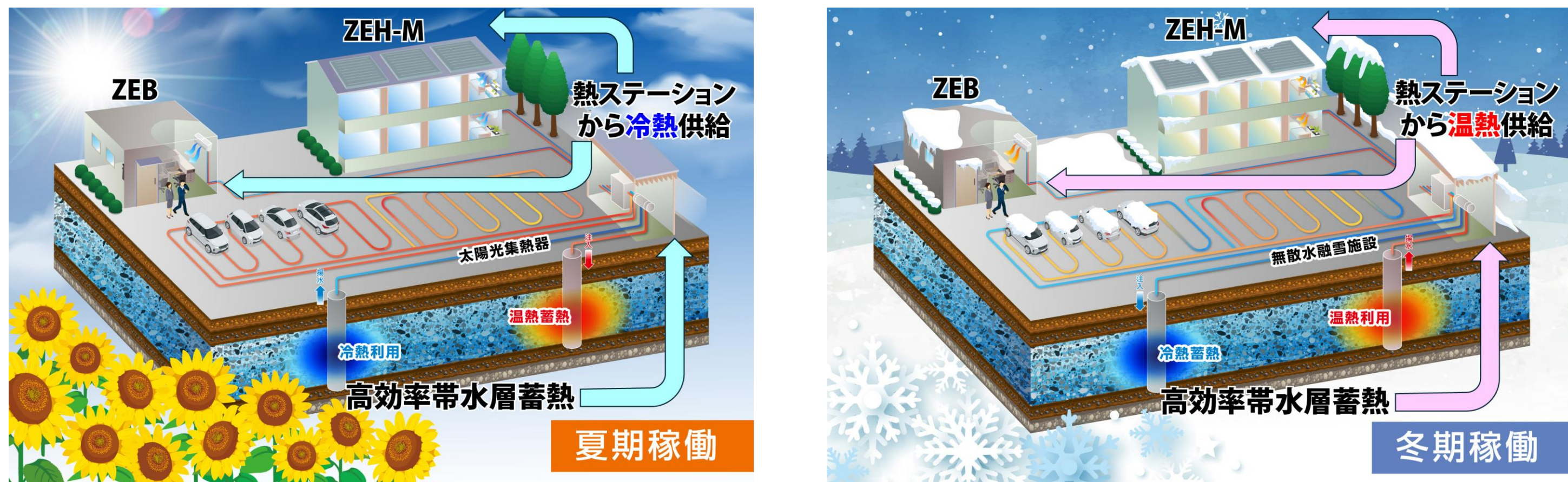
図 帯水層蓄熱を中心とした面的熱利用によるZEB及びZEH-Mの運用イメージ
