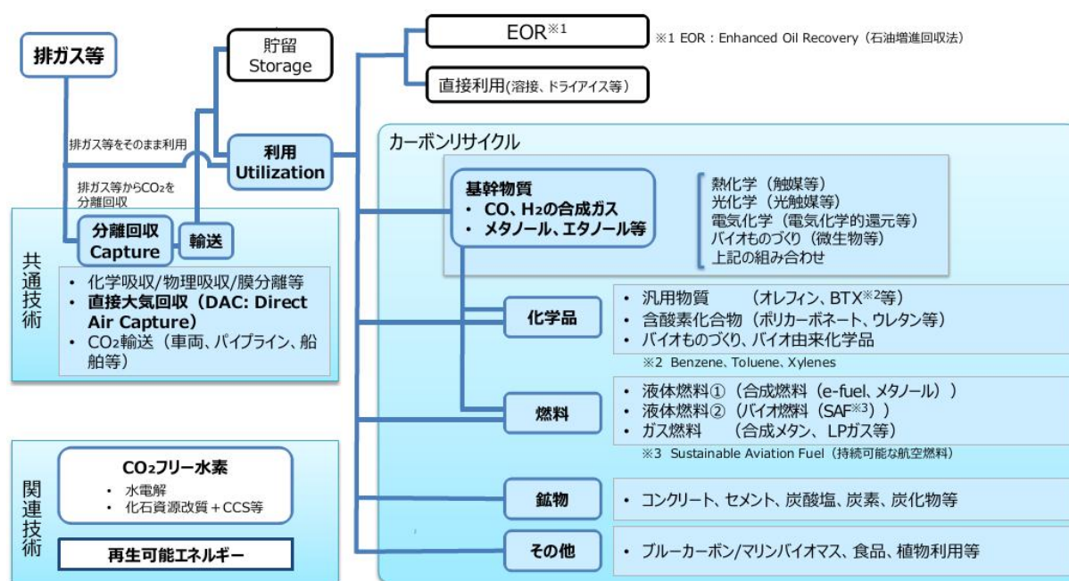
図 1 カーボンリサイクル技術体系図
