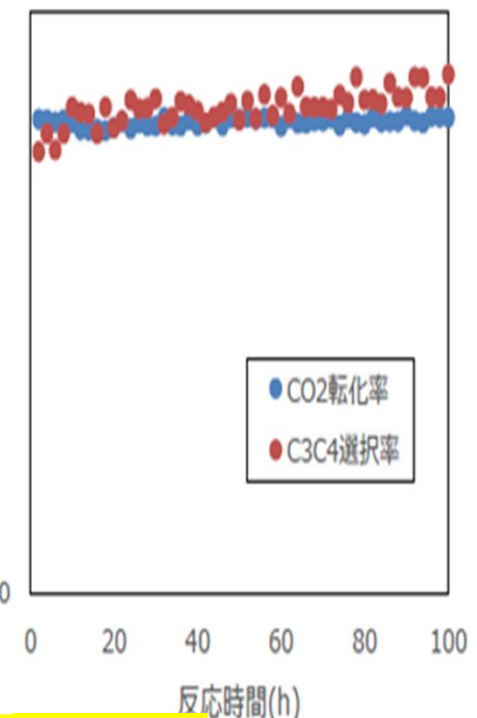
100時間耐久試験実績
