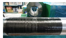
CFRPシリンダーのFW成形
