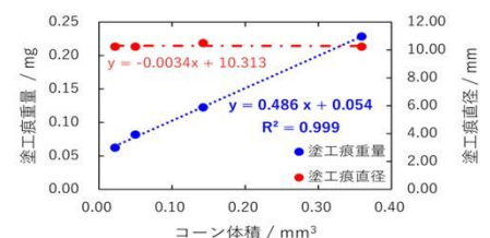
(b) コン体積と塗布痕重量・直径
