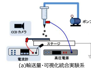
(a) 輸送量・可視化統合実験系
