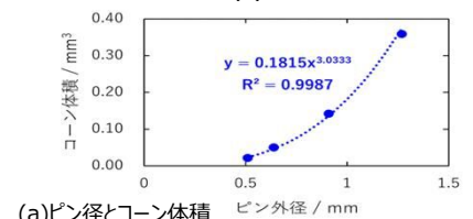
(a) ピン径とコン体積
