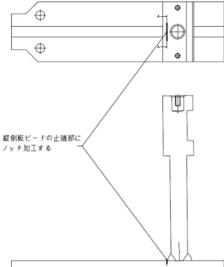
L字構造要素試験体形状
