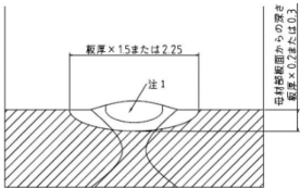
切欠き導入位置
