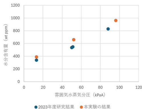
図3 零昇気蒸気分圧とガラス中の水分含水量
