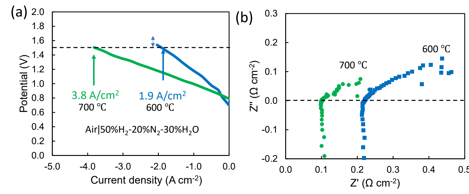
図 作成したNi支持LSGM薄膜セルの電解特性(a)と内部抵抗(b)
