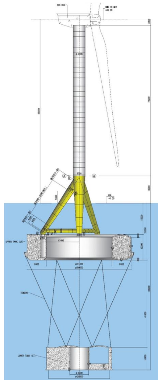
6MW実証機基本図
