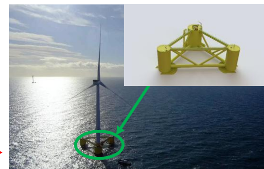
セミサブ型浮体▶
