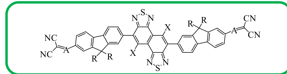
NTz-F-CN
