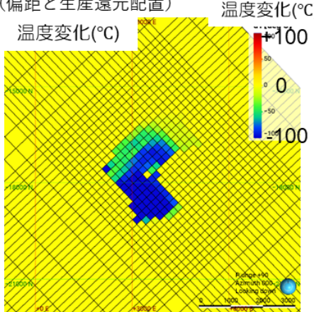
図4：貯留層温度の変化 (最大発電量推定：生産開始30年後)
