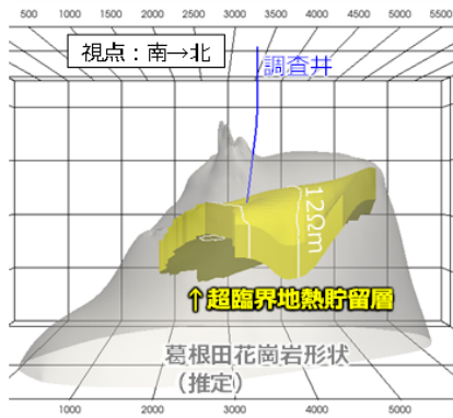
図1：葛根田地域の超臨界地熱貯留層
