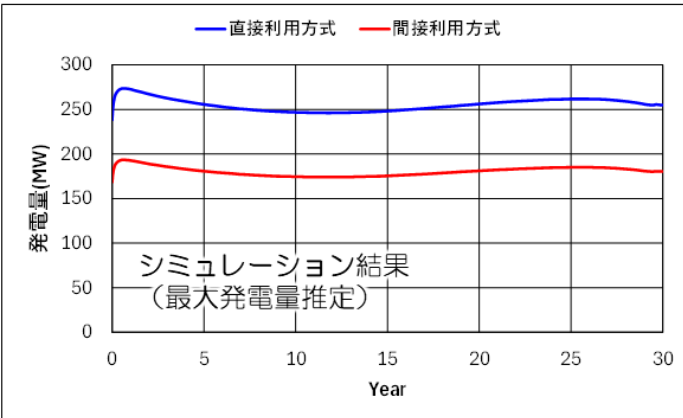
図3：発電量の推移（最大発電量推定）
