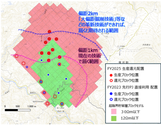
図2：超臨界地熱貯留層数値モデル (偏距と生産還元配置)
