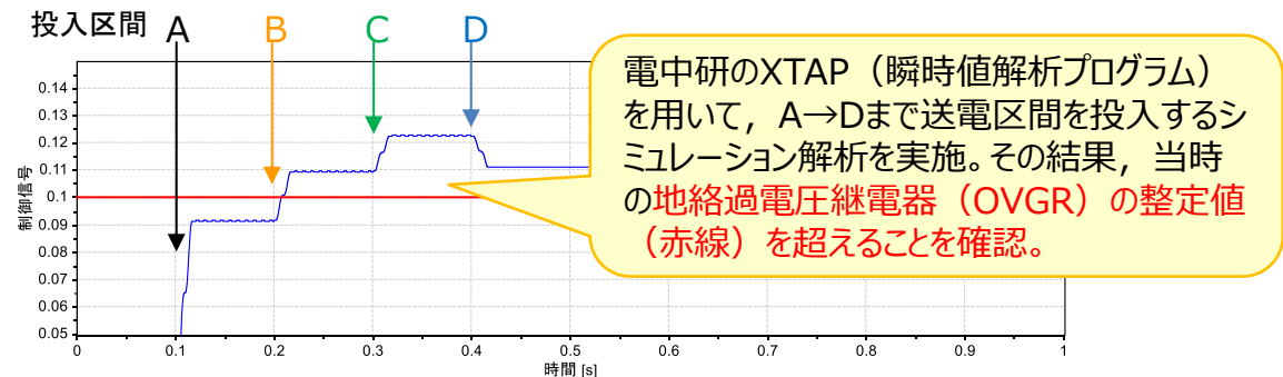
零相電圧のシミュレーション結果
