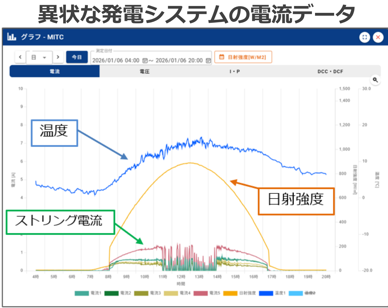
電流・日射・気温の時系列データ
