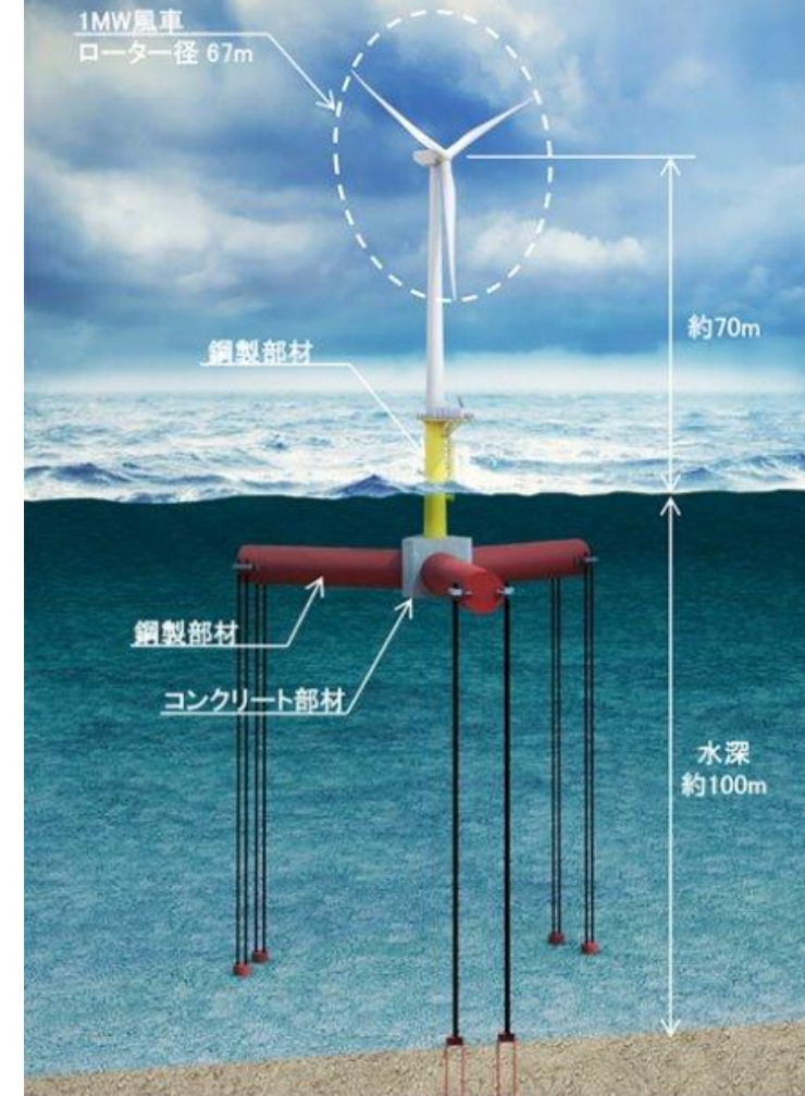
1MW風車搭載浮体
