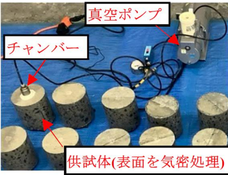
透気試験状況
