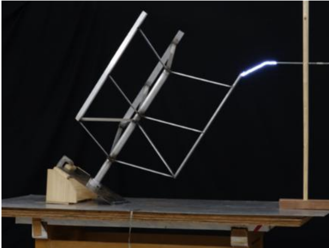
高電圧試験における着雷の瞬間
