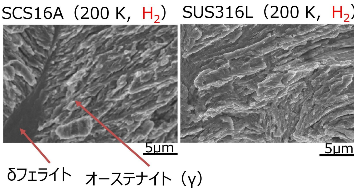
δフェライト オーステナイト (γ) オーステナイトの破面は SUS316Lに類似
