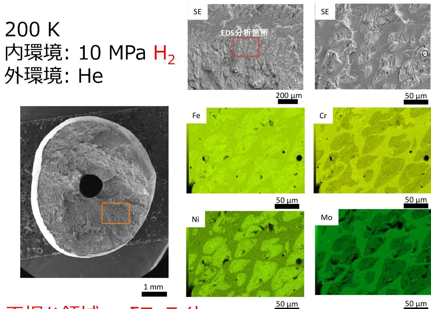
平坦な領域・・・δフェライト 凹凸のある領域・・・オーステナイト 200 K 内環境: 10 MPa H_2 外環境: He 水素暴露側の破面ではδフェライトを観察
