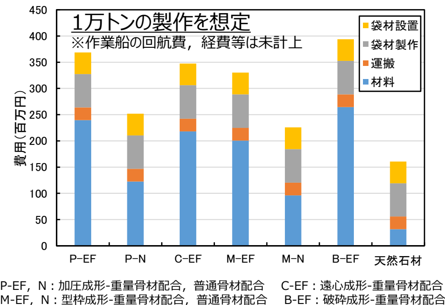
袋型根固め材（袋材）の製作・設置費試算 （直接工事費のみ）
