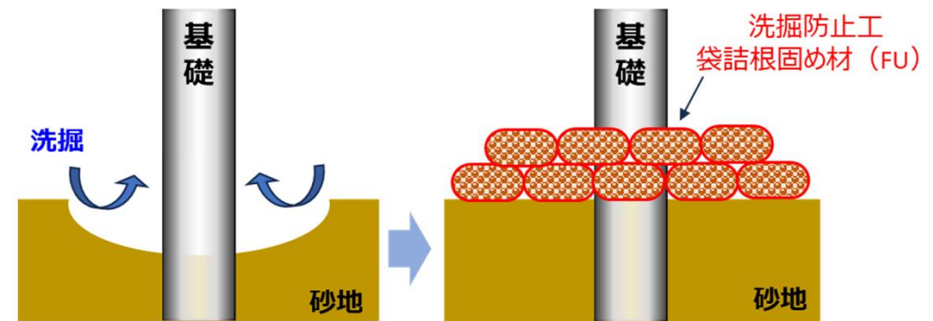
モノパイル基礎部の洗掘防止
