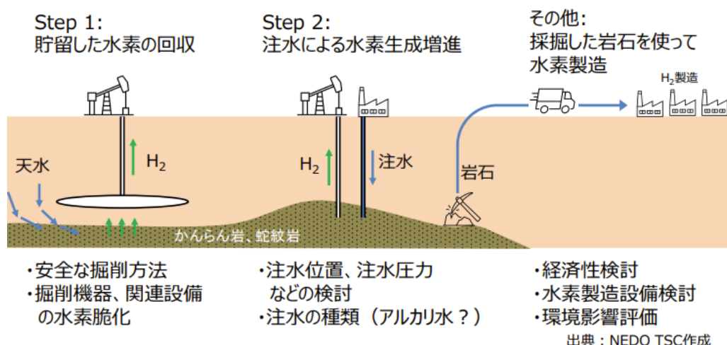
図 1-20 天然水素回収・生産増進プロセス 171
