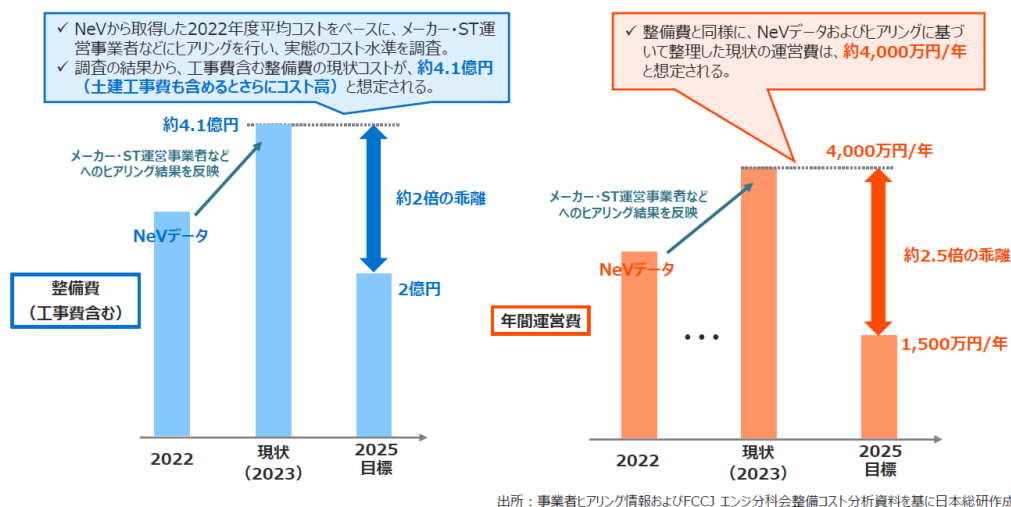
図 1-24 LDV 向け水素ステーションの整備費・運営費目標と現状とのギャップ分析 182
