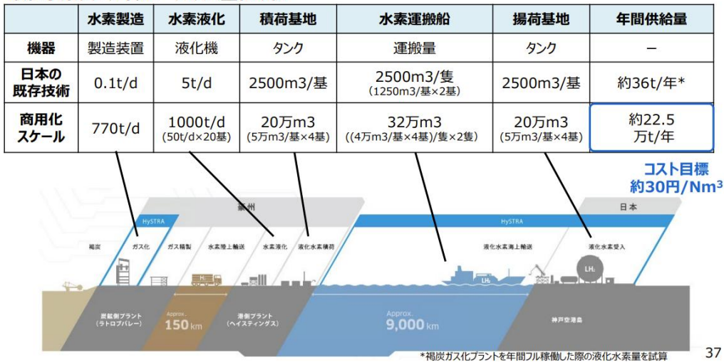
図 1-9 液化水素サプライチェーンにおける現状の主要機器性能と商用規模の例 105
