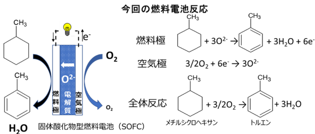
図 1-15 SOFC による MCH 直接発電技術概要 138
