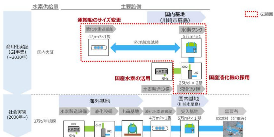
図 1-8 GI 基金事業「液化水素サプライチェーンの商用化実証」におけるサプライチェーン概要 114
