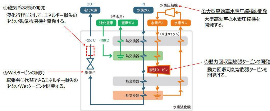
図 1-13 液化技術システム概要及び技術開発テーマ 134
