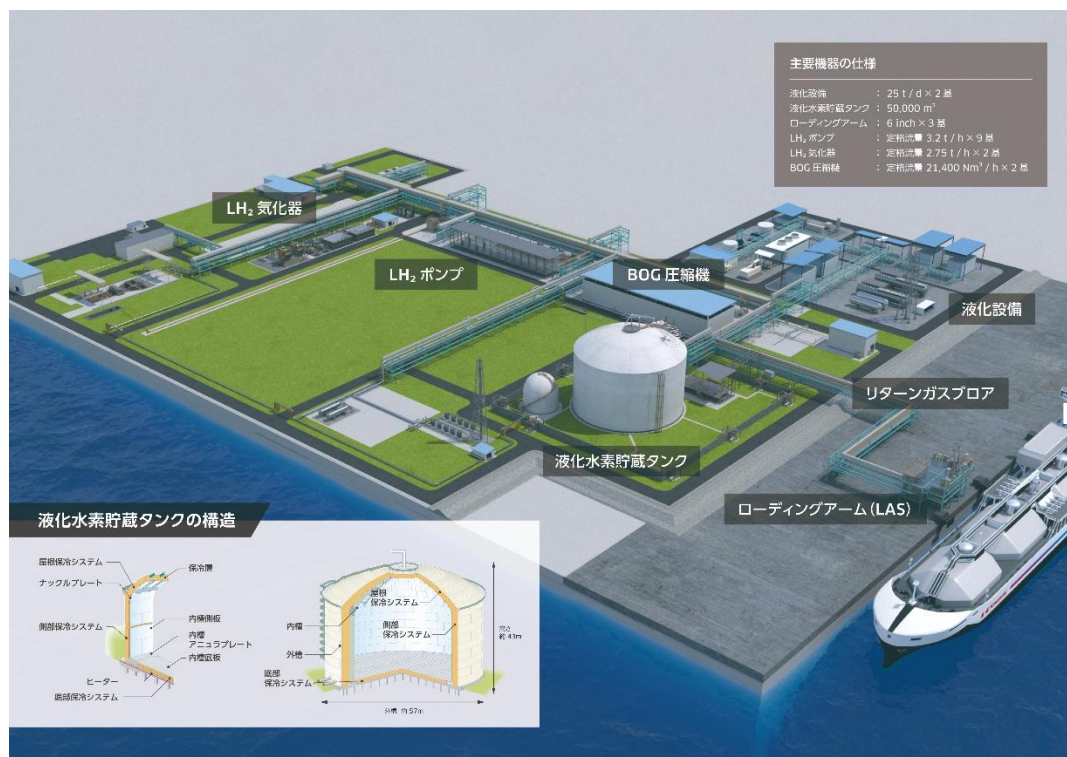
図 1-10 「川崎 LH 2 ターミナル」の完成イメージと設置予定の 5 万 m 3 液化水素貯槽タンクの構造 129
