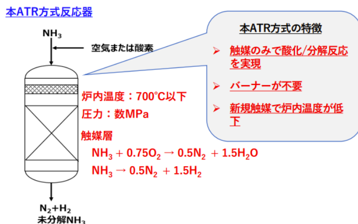
図 1-17 オートサーマル方式の概要 155
