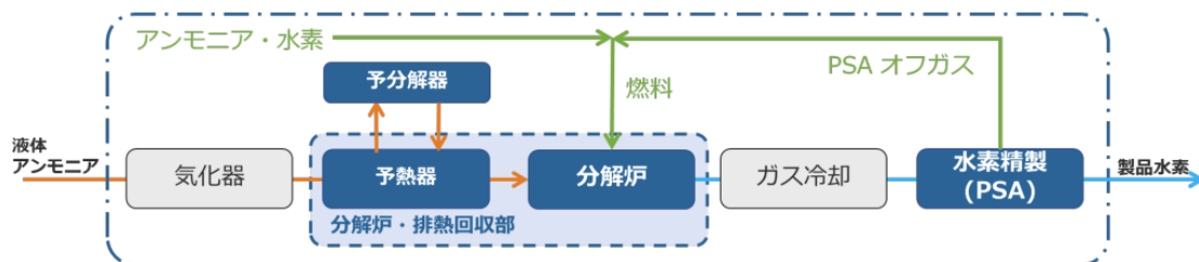
図 1-16 ファーネス方式（大規模外部加熱分解）のシステム概要図 151
