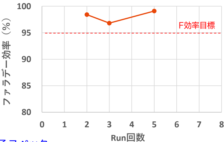
DSS運転時のファラデー効率推移(@6kA/m 2 )
