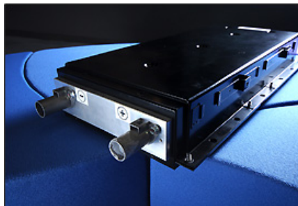
日立ビークルエナジーのハイブリッド自動車用量産型リチウムイオン2次電池セル（左）。セルを48本直列した製品モジュール（右）。乗用車ならモジュール一つ、トラックのような大型車では、モジュール二つをつなげて使用する。
